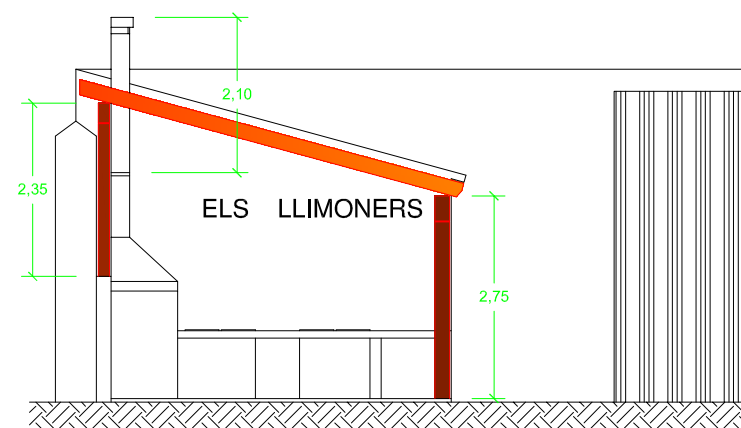
ALÇAT LATERAL
